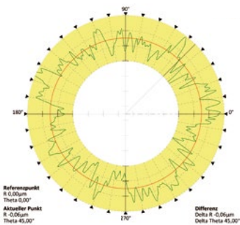
Rundheit vor Microfinish
