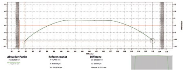
Profil nach Microfinish
