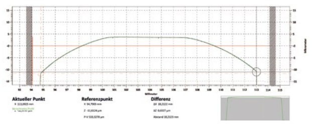
Perfil após microacabamento
