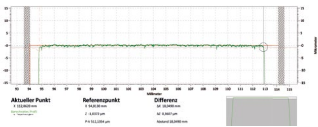
Perfil antes do microacabamento
